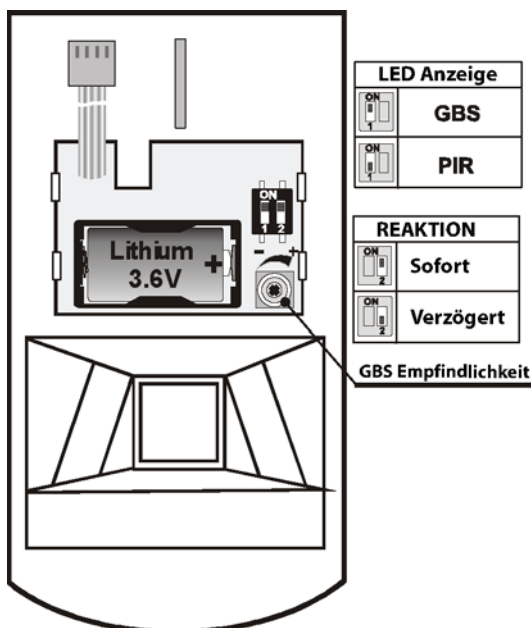
Glasbruchmelder
