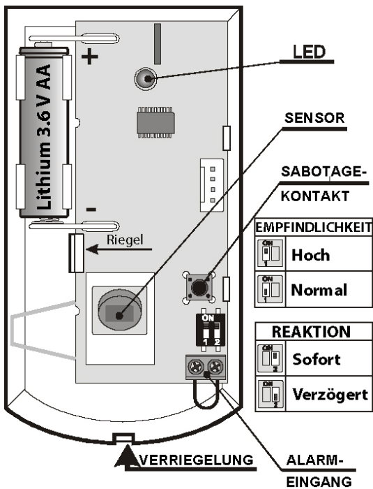
PIR-Bewegungsmelder
