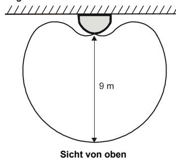
Erfassungsbereich des Glasbruchmelders
